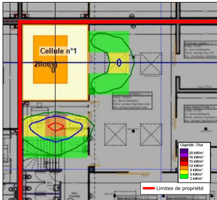
Figure 2. Représentation graphique effets thermiques générés par un incendie sur le stockage frigorifique de matières premières
